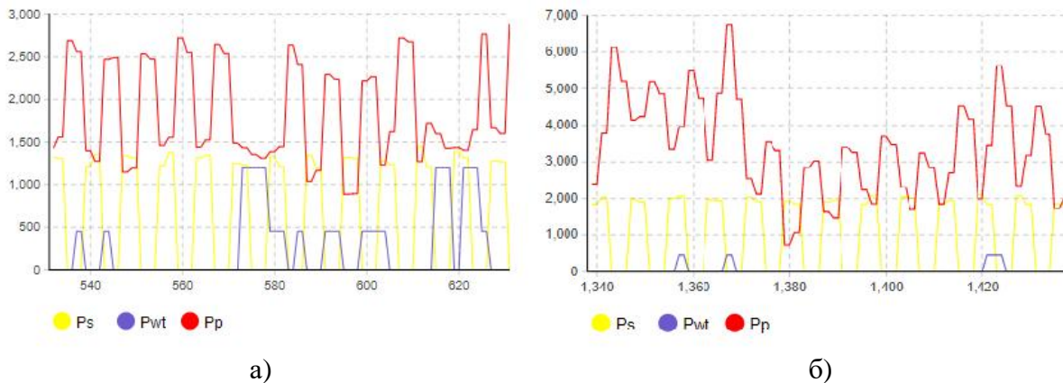
Рис. 3. Графики электроэнергии для варианта 1: а) для марта; б) для июля
