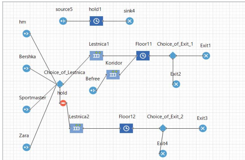
Рис.1. Имитационная модель плана ТЦ в AnyLogic
