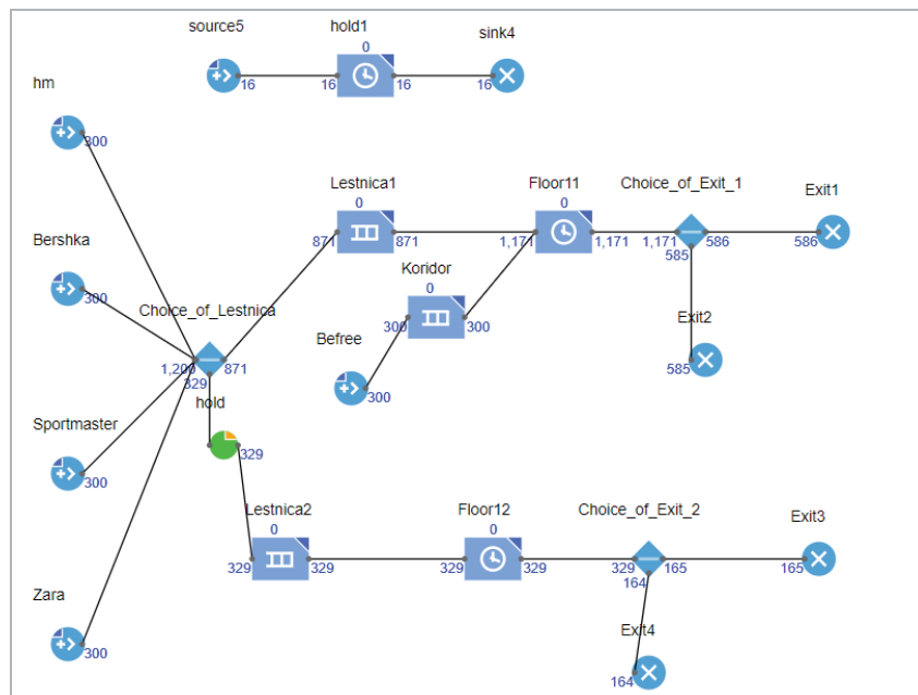
Рис.2. Имитационная модель плана ТЦ в AnyLogic после запуска
